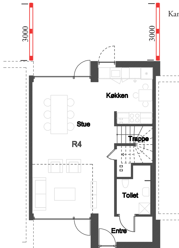
STUEPLAN
